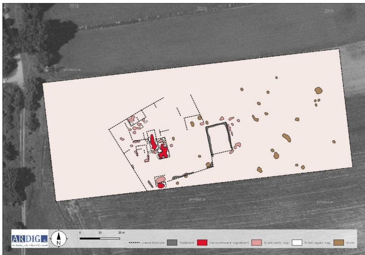
Abbildung 4: Interpretation der geophysikalischen Messergebnisse. (Quelle: Fa. ARDIG, GmbH)
